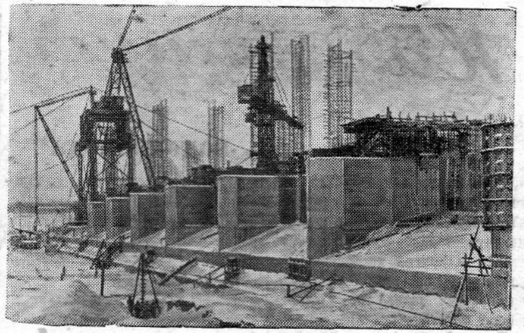
Недалеко от города Горького, на Волге возводится Горьковская гидроэлектростанция. На снимке: общий вид строительства водосливной плотины.
