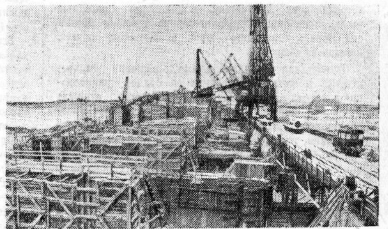
На снимке: общий вид строительства водосливной плотины Новосибирской ГЭС. Бетонные работы ведутся здесь безостановочно всю зиму и даже в самые лютые морозы в закрытых, обогреваемых паром, блоках. Фото В. Лещинского. Фотохроника ТАСС.
