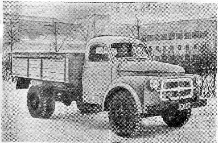
ГОРЬКИЙ. Коллектив Горьковского автозавода имени В. М. Молотова изготовил опытный образец грузового автомобиля «ГАЗ-52», который в недалеком будущем заменит ныне выпускаемый грузовой автомобиль «ГАЗ-51». Новая машина будет расходовать горючего на 12—15 процентов меньше. На ней установлена коробка перемен передач с синхронизатором, что значительно облегчит управление. Новый автомобиль имеет рессорную подвеску на резиновых подушках. На снимке: новая опытная грузовая автомашинка «ГАЗ-52». Фото В. Храмова. Фотохроника ТАСС.
